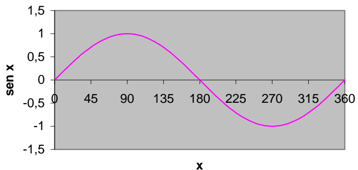
Gráfica de la función seno
