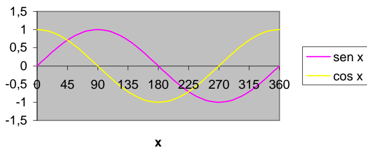
Gráficas del seno y coseno
